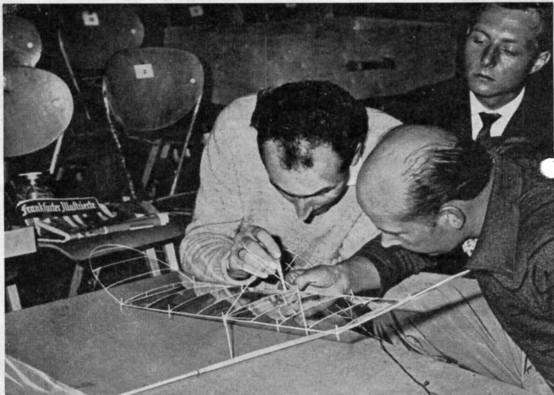
Karl-Heinz Rieke, Berlin, startet sein 90-cm-Mikrofilm-Modell. Es hat 1,4 g Zellengewicht.
