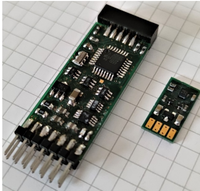
PK-400 mit Sensorplatine PK-400 with sensor board
